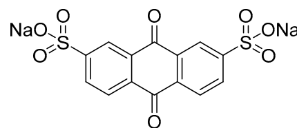
2,7-AQDS disodium salt aqueous solubility: 0.58 / 0.74 M
