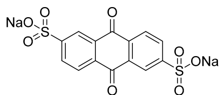
2,6-AQDS disodium salt aqueous solubility: 0.04 M
