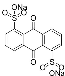
1,5-AQDS disodium salt aqueous solubility: 0.07 M
